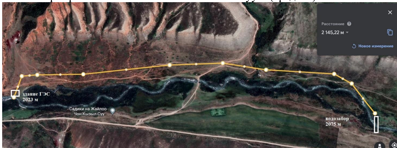
Рис. 3. Карта расположения МГЭС Чон-Кызыл-Суу-2 (средняя).
