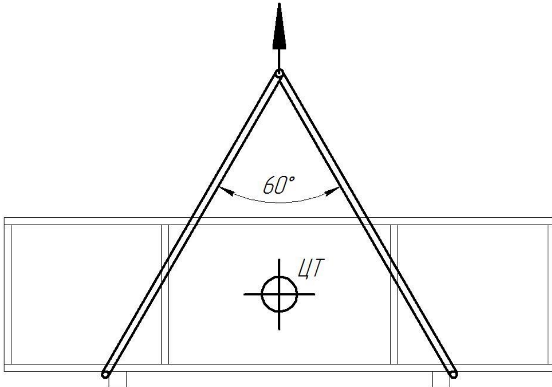
Рисунок 8 – схема строповки ящика с измерительным компонентом устройства I-TOR-35.
