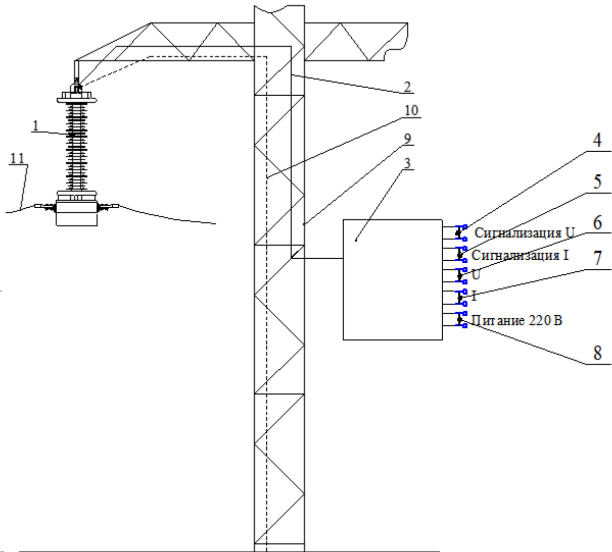
Рисунок 1А. Блок – схема устройства I-TOR-35 (на примере измерительного компонента, выполненного в виде подвесной конструкции)
