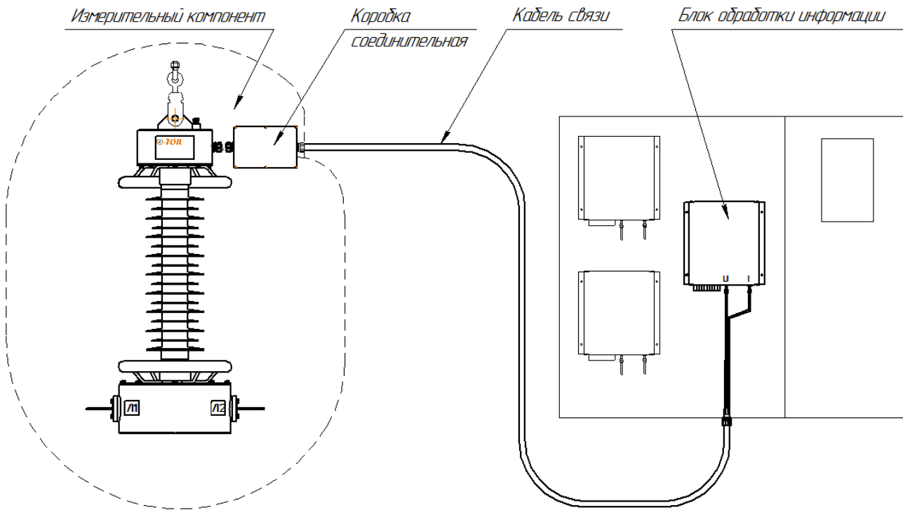
Рисунок 1Б. Структурная схема I-TOR-35 (на примере измерительного компонента, выполненного в виде подвесной конструкции)
