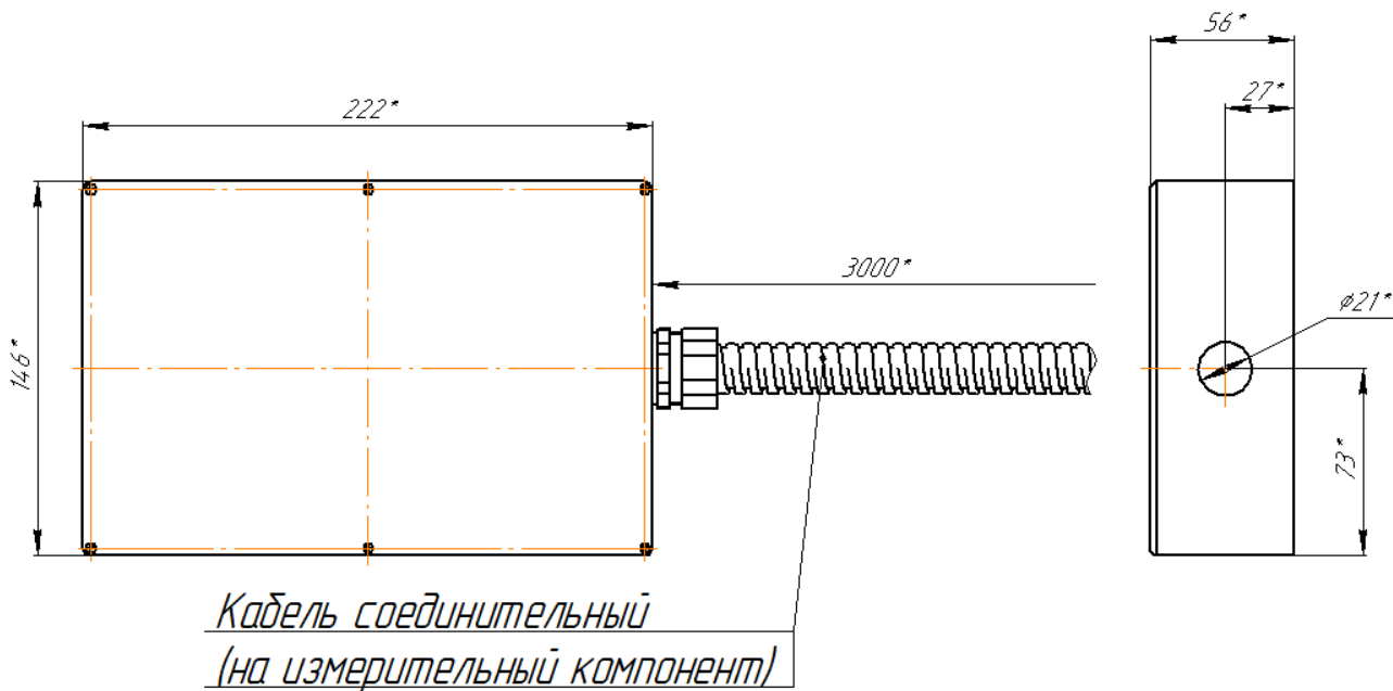
Рисунок 2Ж – габаритно-установочные размеры коробки соединительной.
