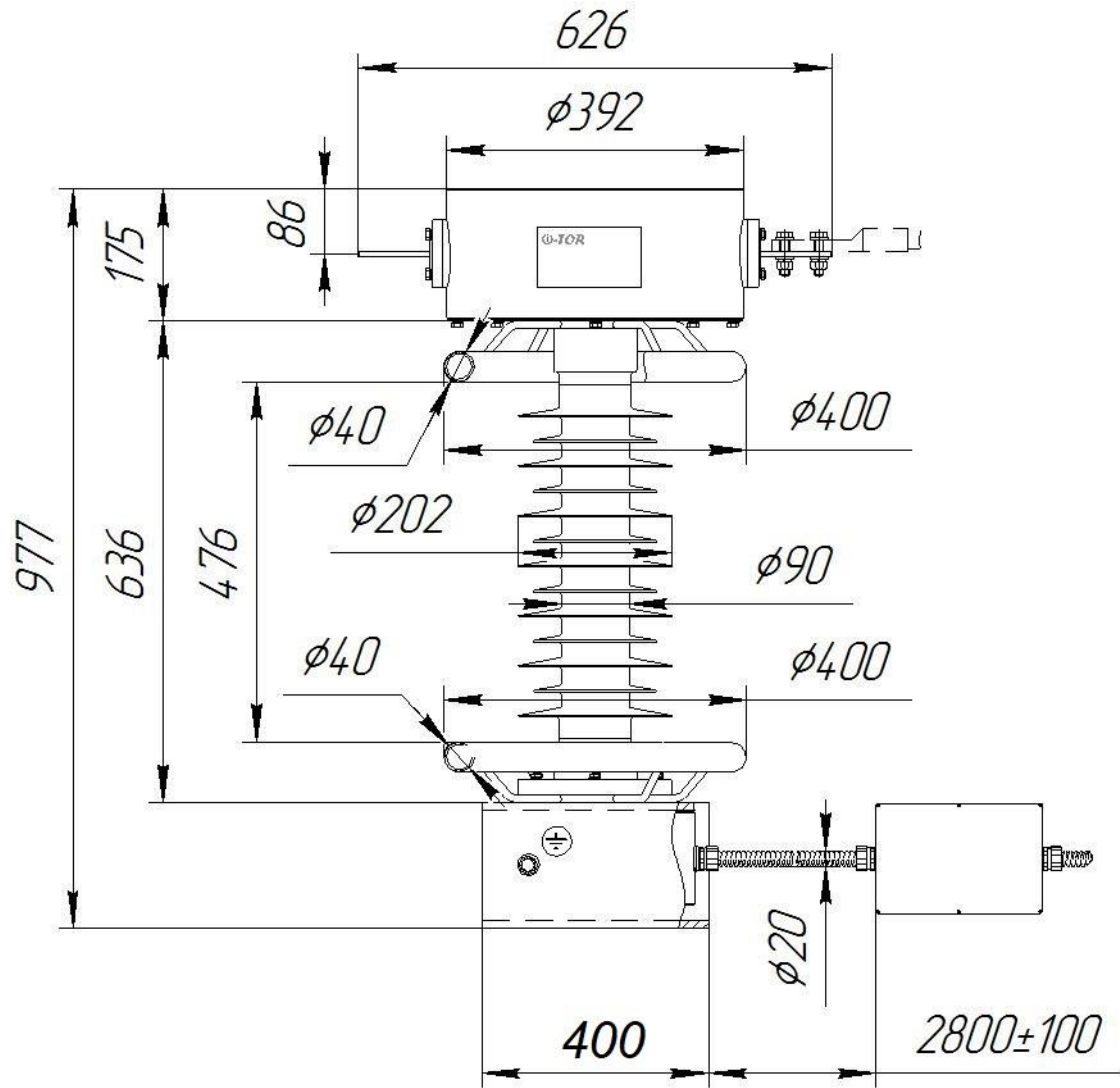
Рисунок 2Б – габаритно-установочные размеры измерительного компонента I-TOR-35, выполненного в виде опорной конструкции. Размеры элементов – места заземления, место для присоединения аппаратного зажима показаны на рисунках 2В, 2Д.
