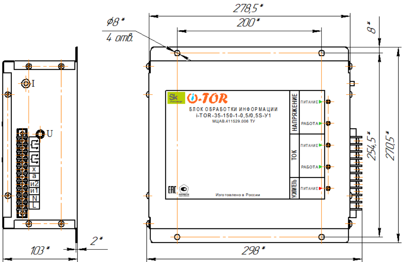
Рисунок 2Е – габаритно-установочные размеры блока обработки информации I-TOR-35
