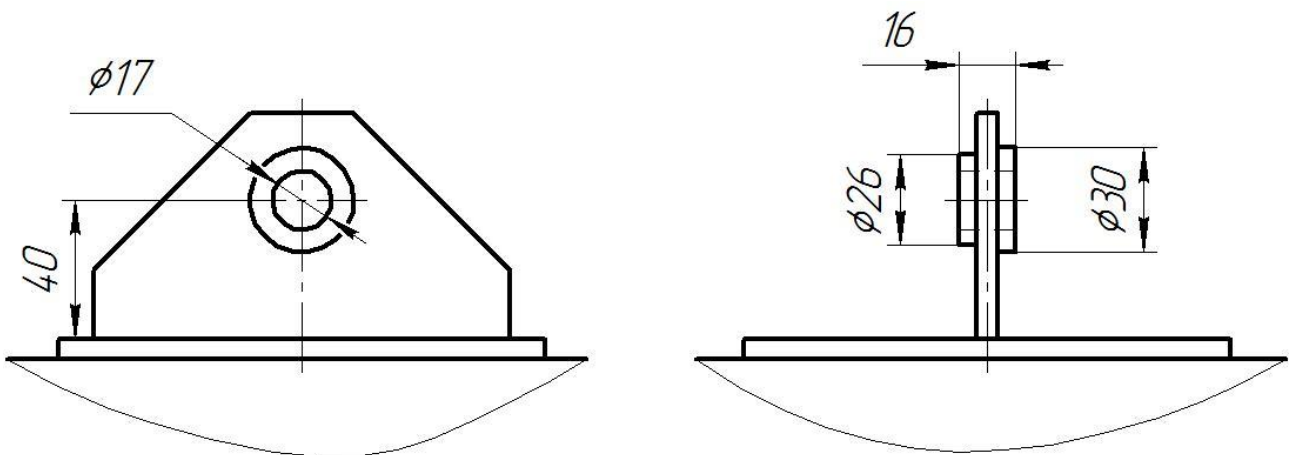
Рисунок 2Г – место подвешивания измерительного компонента I-TOR-35
