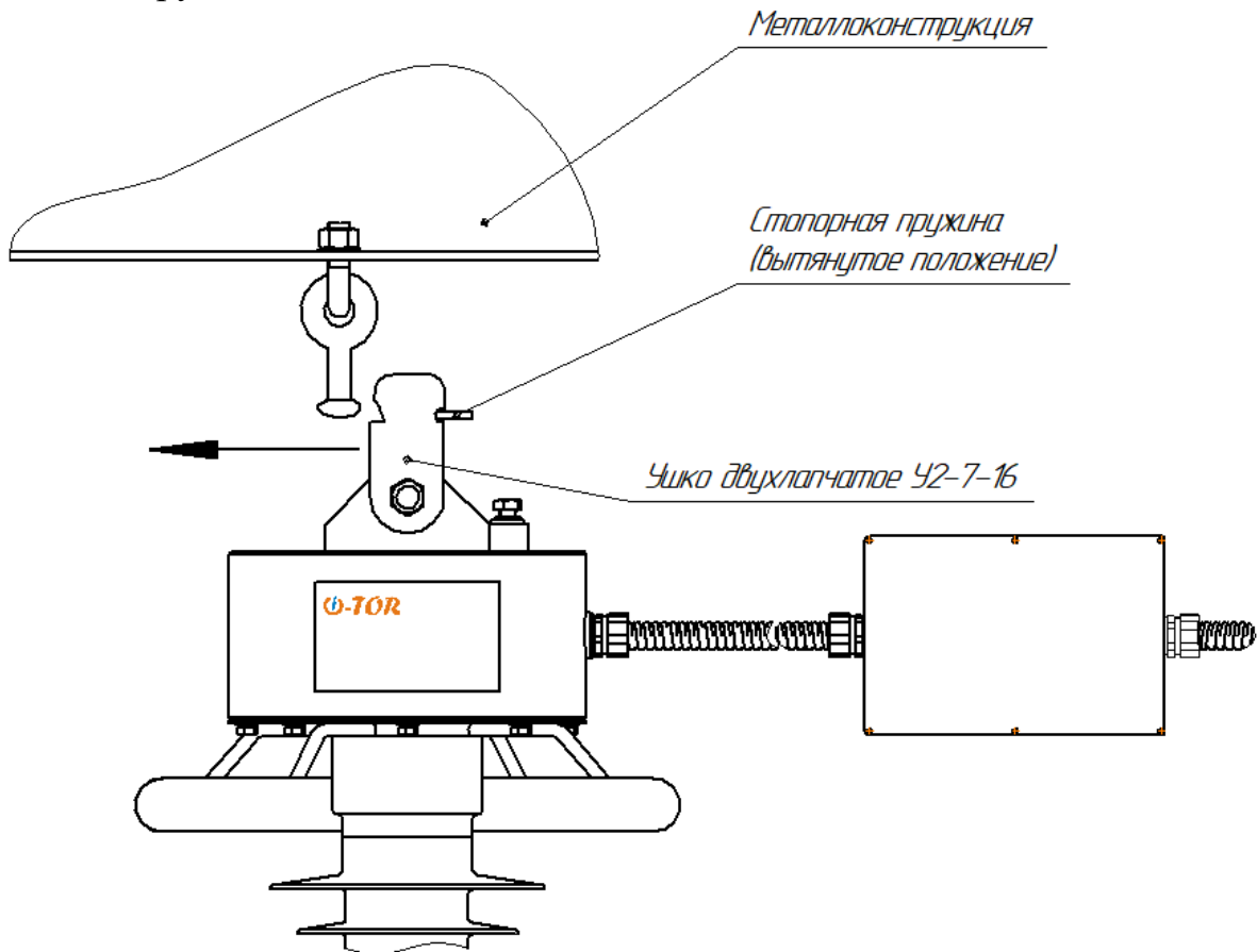
Рисунок 4 – смыкание элементов подвеса
